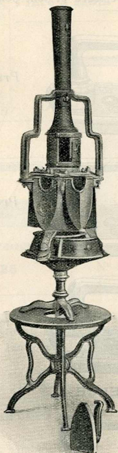
Appareil N° 9 muni du Cendrier-Tiroir
